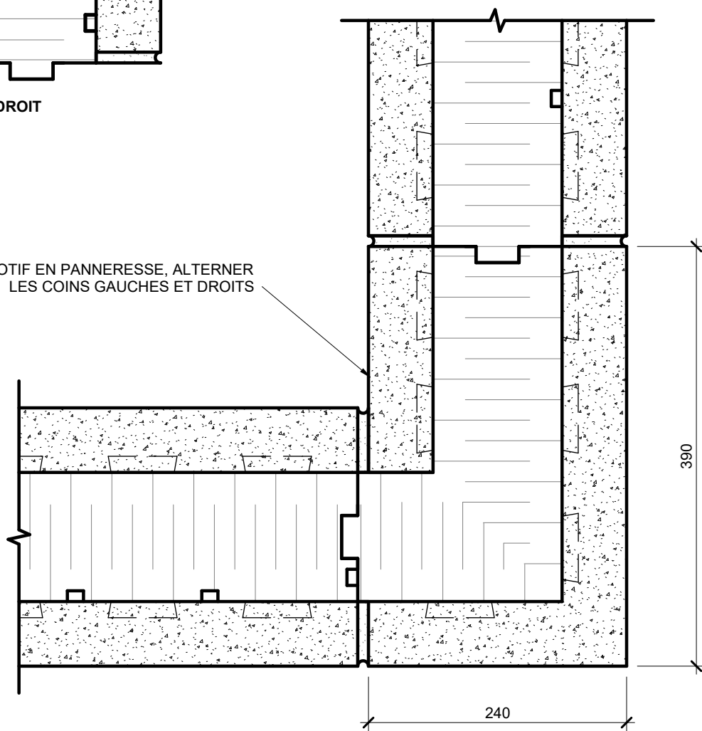
DÉTAIL TYPE - BLOCS DE COIN
